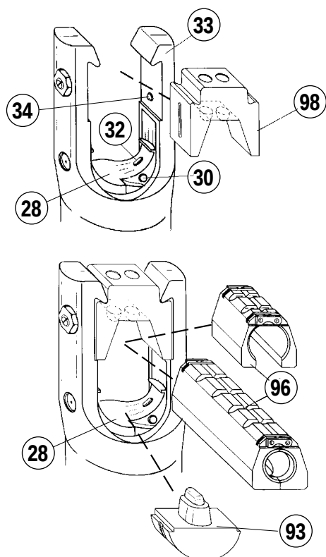
FIG. 5 DIES REPLACEMENT / INSERTION DES MATRICES / EINRASTEN PRESSEINSATZE INSERCIÓN DE LAS MATRICES / INSERIMENTO MATRICI
