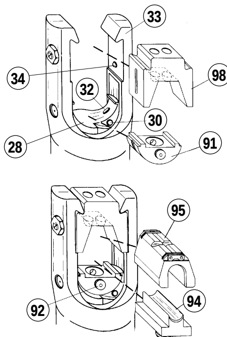
FIG. 5 DIES REPLACEMENT / INSERTION DES MATRICES / EINRASTEN PRESSEINSATZE INSERCIÓN DE LAS MATRICES / INSERIMENTO MATRICI
